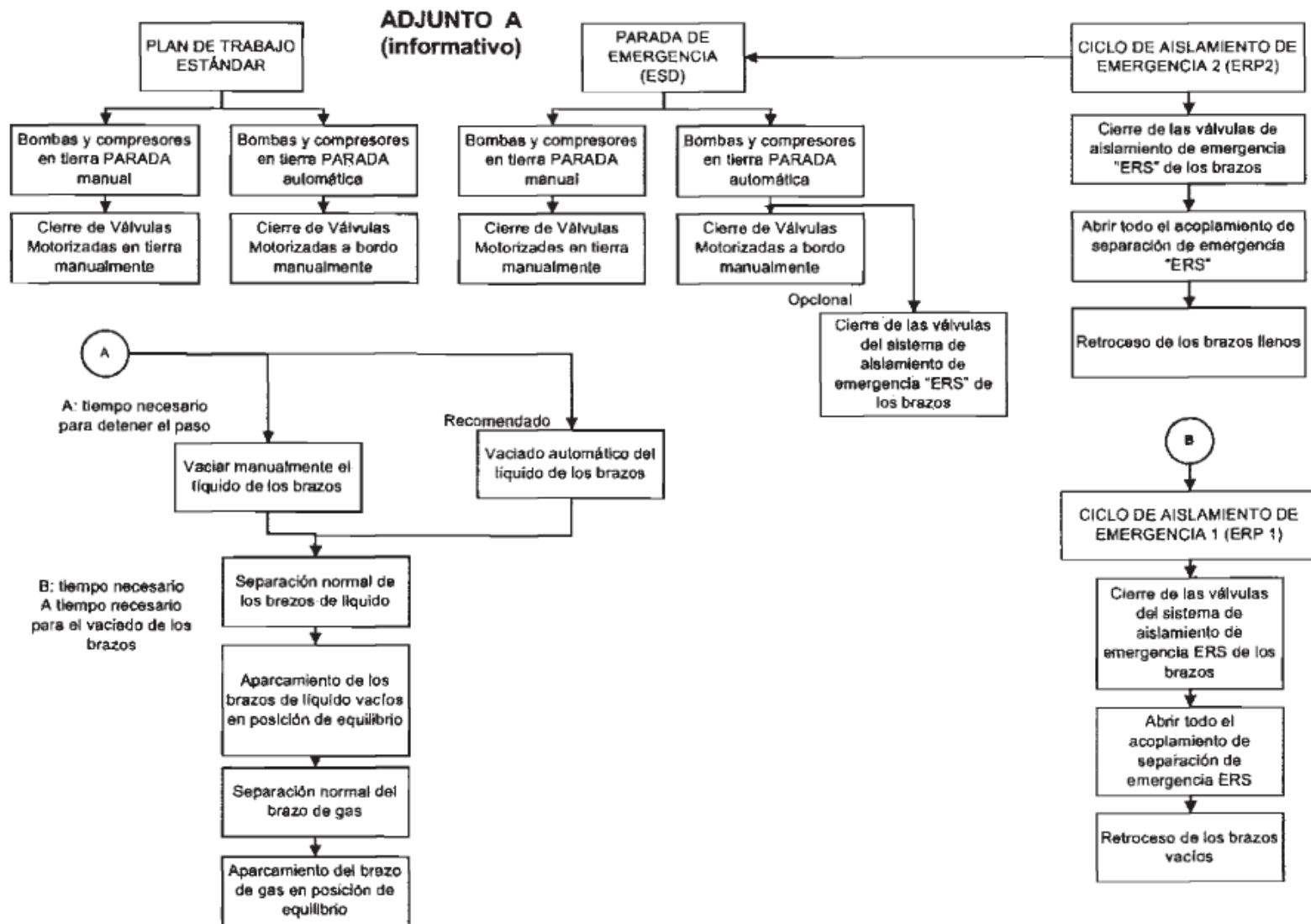
Fig A1 – concepto general de seguridad para detener la carga y descarga de gas licuado
