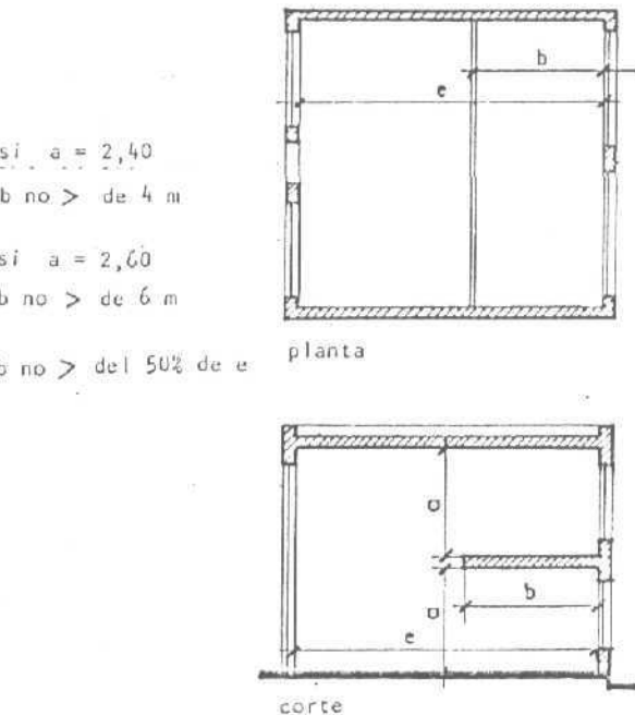
ESQUEMA 3.4.2.3. (a) Entrepisos en negocios
