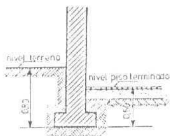
ESQUEMA 4.5.1.2. b) corte
