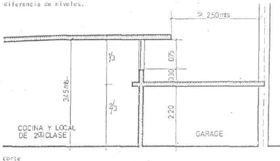
ESQUEMA 3.4.4.2. (d) Ventilación de locales de 2da. clase por diferencia de niveles.
