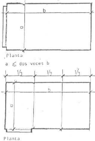
ESQUEMA 3.4.4.2. (b) Iluminación y ventilación de locales 1ra. y 2da. clase que sean profundos
