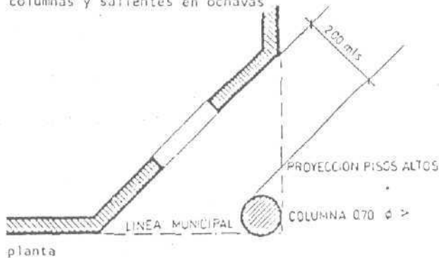
ESQUEMA 3.3.2.8. columnas y salientes en ochavas
