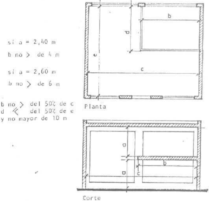
ESQUEMA 3.4.2.3. b) Entrepisos en negocios
