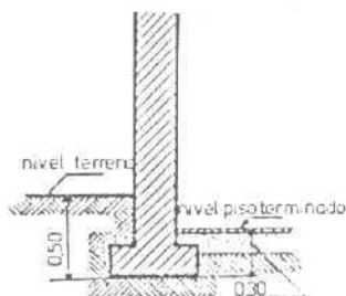
ESQUEMA 4.5.1.2. a) corte
