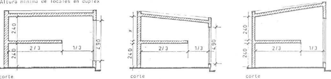
ESQUEMA 3.4.2.3. Altura mínima de locales en duplex
