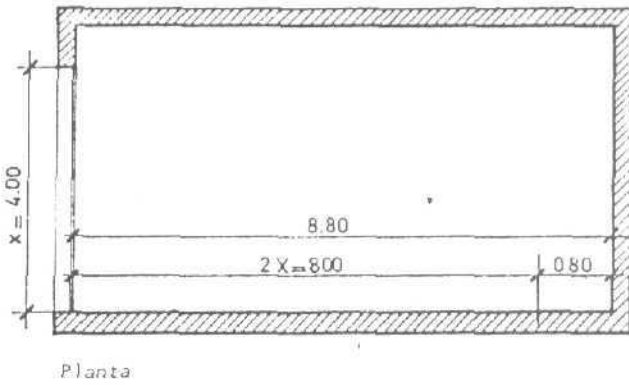
ESQUEMA 3.4.2.5. Relación de altura con profundidad
